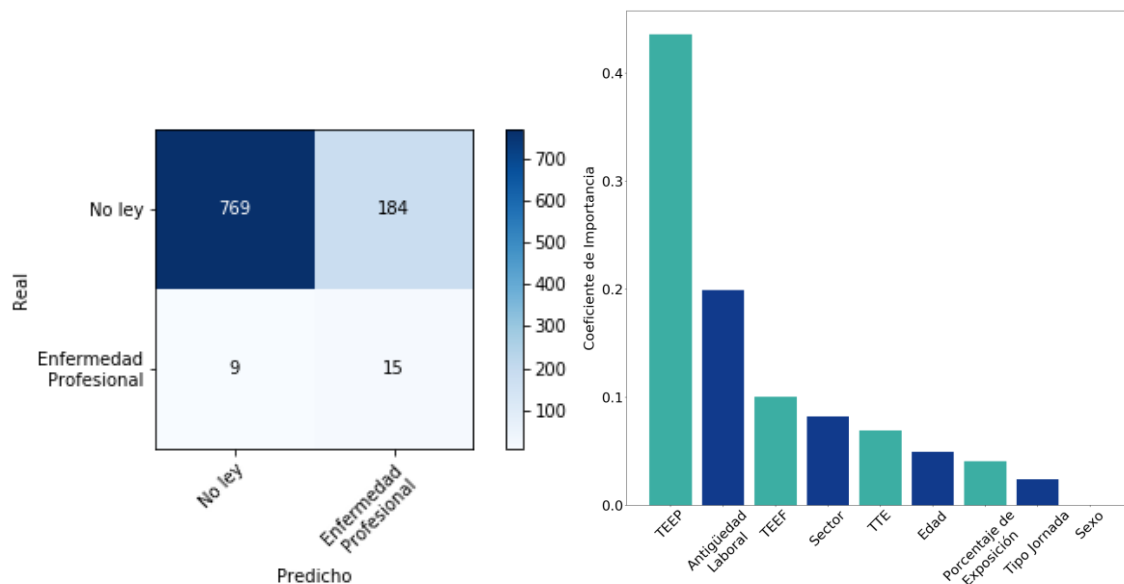
Figura 16. Matriz de confusión y lista de importancia de variables. En la figura se muestra el rendimiento de clasificador con la partición de test la base de datos (977 sinistros) en la matriz de confusión (izquierda) y la importancia de las variables para el mismo clasificador (derecha).
